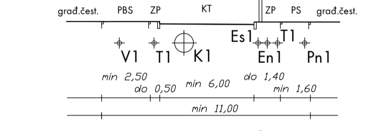
UK2 - presjek 2-2
