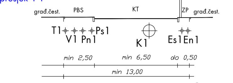
UK1 - presjek 1-1
