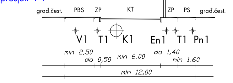
UK4 - presjek 4-4
