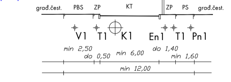
UK3 - presjek 3-3
